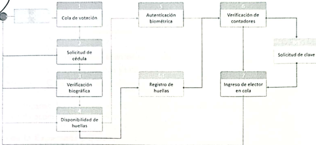
Workflow de autenticación
